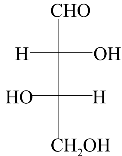
L-Threose
