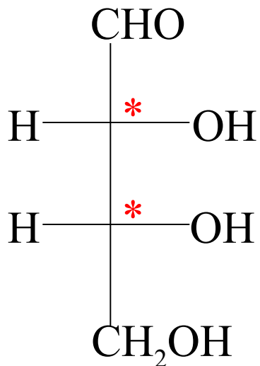
D-Erythrose
