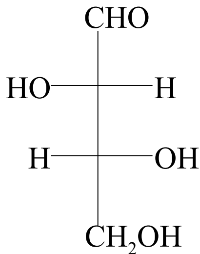
D-Threose
