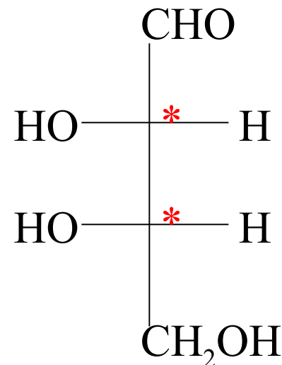
L-Erythrose
