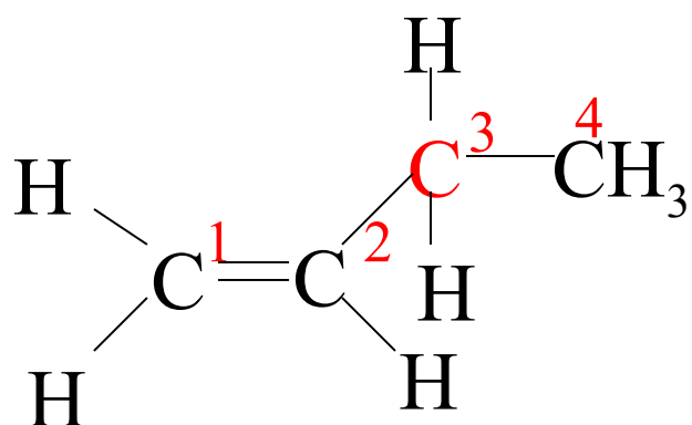
1-butene
