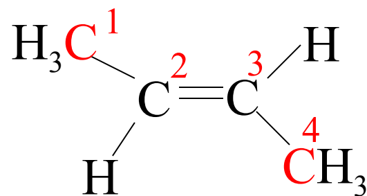
trans -2-butene
